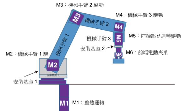
< 機器人構成示意圖 (從側面) >
