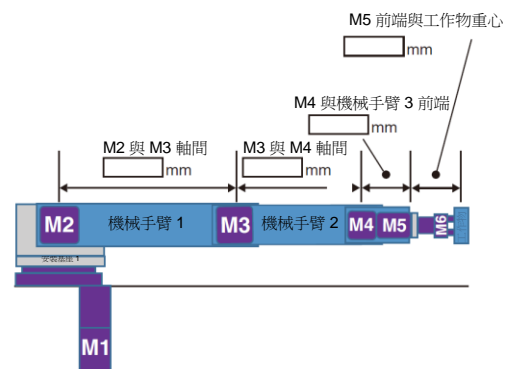
< 機器人構成示意圖 (從側面) >
